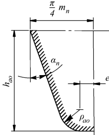
Fig. 4.2.2.7.3.2-2. Non-protuberance hob Fig. 4.2.2.7.3.2-3. Non-protuberance hob
